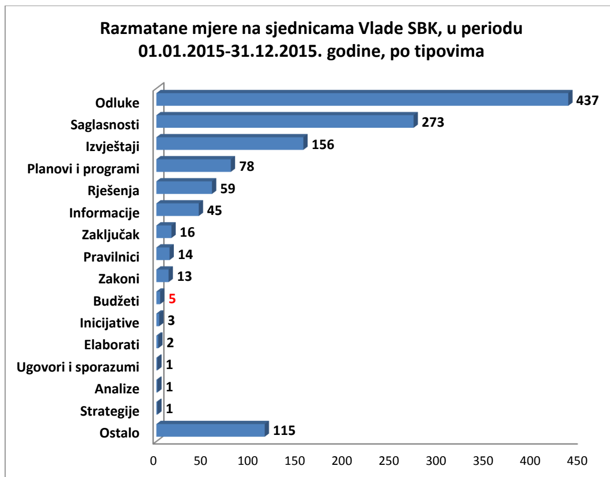
Grafikon 4
