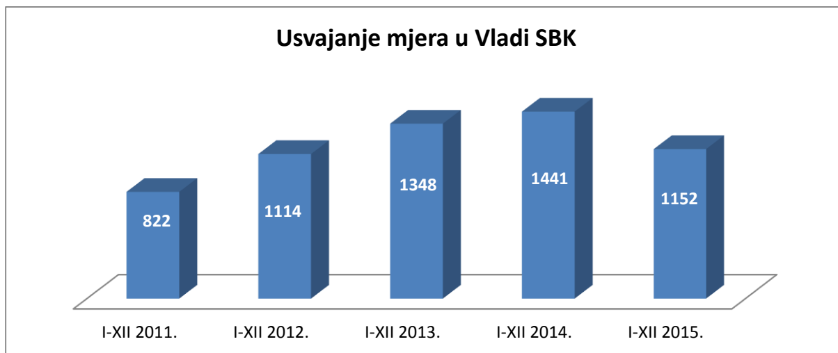
Grafikon 8
