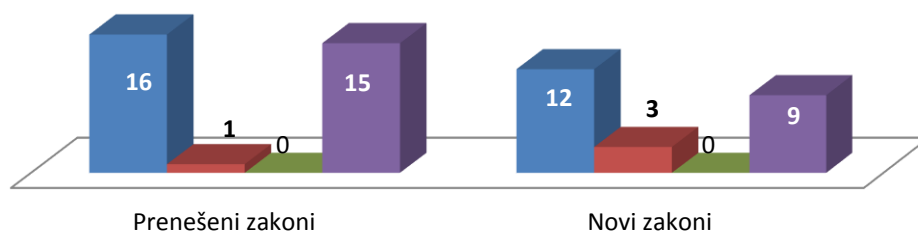
Grafikon 18
