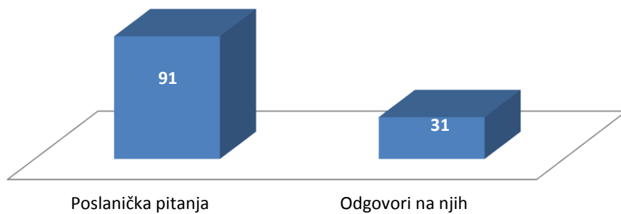
Grafikon 29
