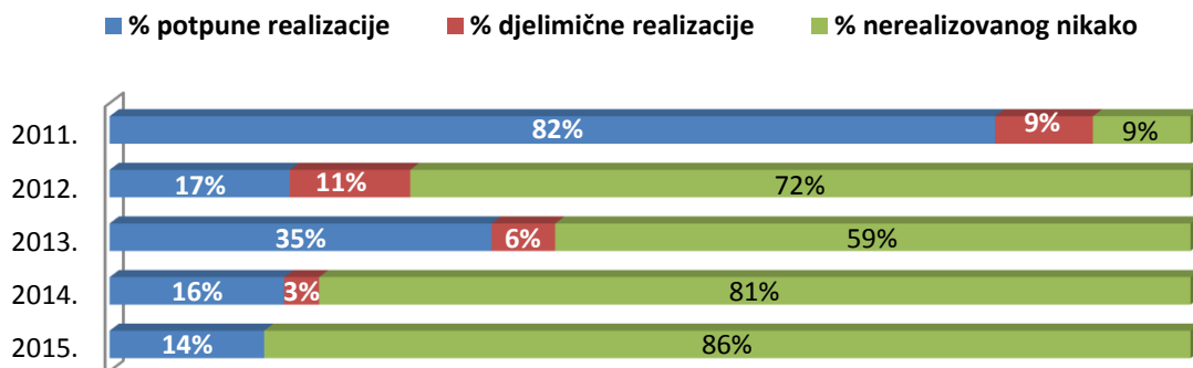
Grafikon 17
