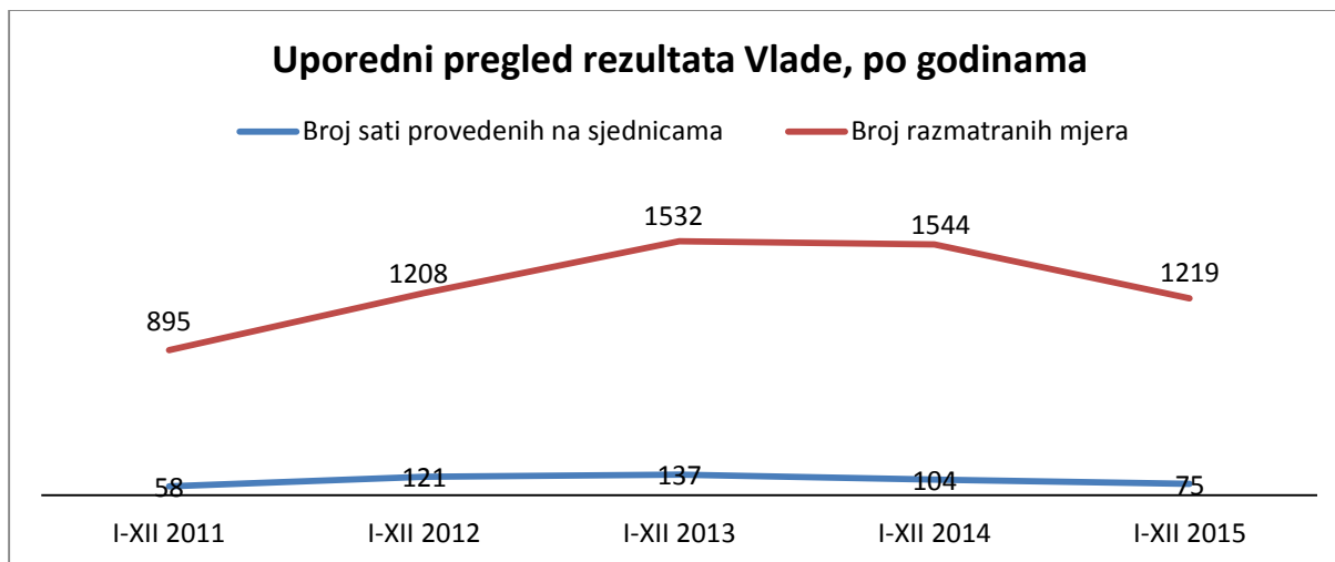
Grafikon 6
