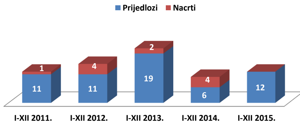
Grafikon 25
