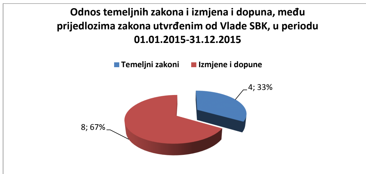
Grafikon 24
